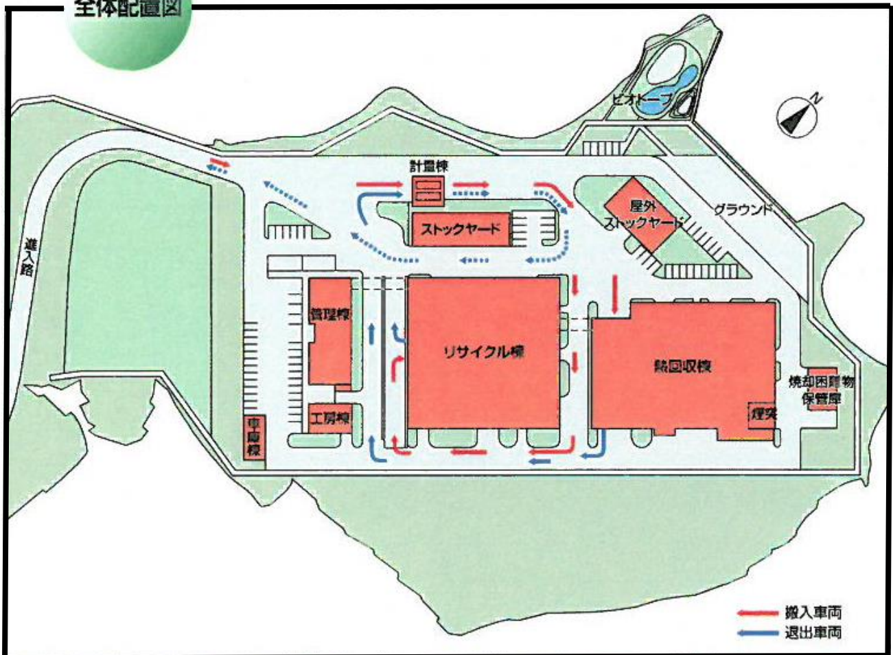
全体配置図
