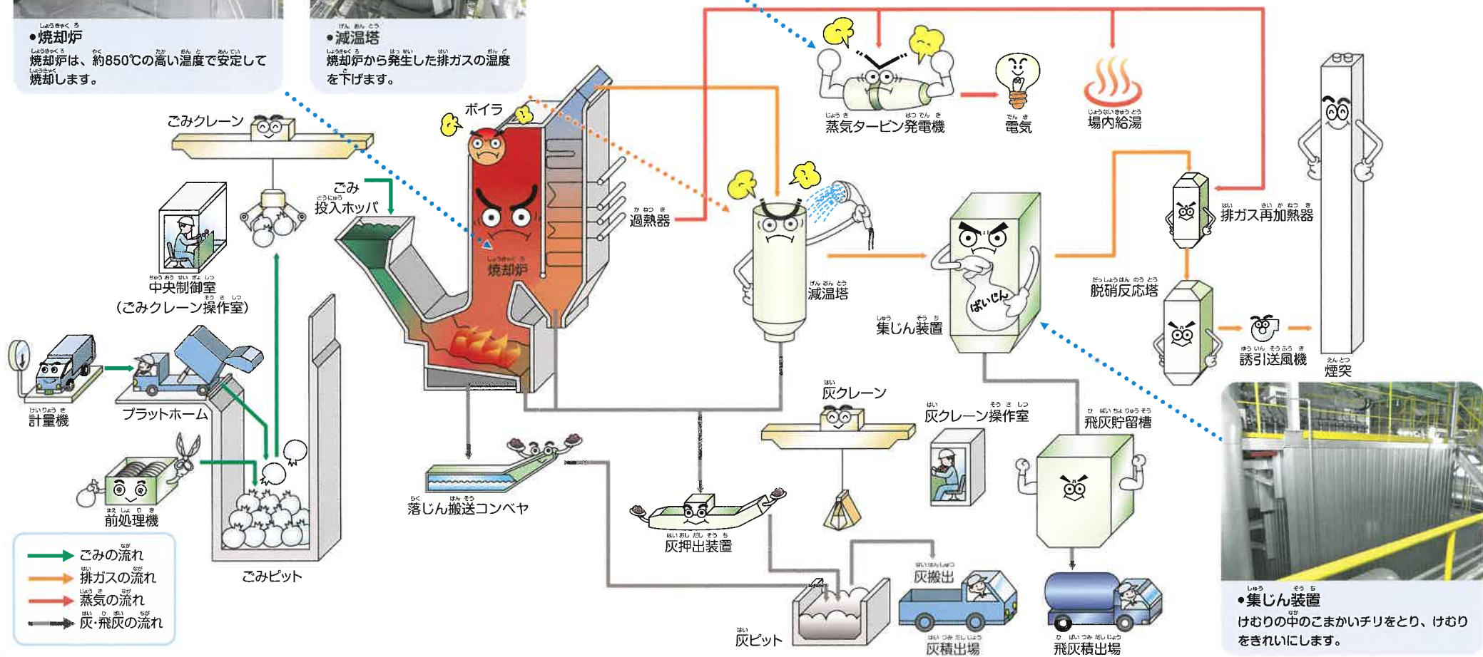
●蒸気タービン発電機 ボイラによって蒸気をつくり、タービン発電機によって電気をつくります。
